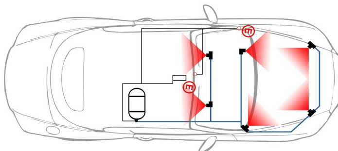
СХЕМА УСТАНОВКИ СИСТЕМЫ ПОЖАРОТУШЕНИЯ В АВТОМОБИЛЕ
